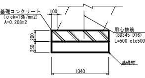
基礎工(750型) S=1:75
