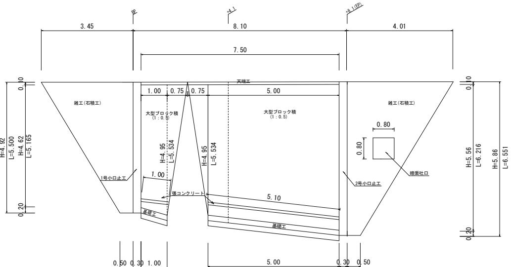
大型ブロック積工展開図 S=1:50
