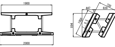
大型ブロック図 S=1:75
