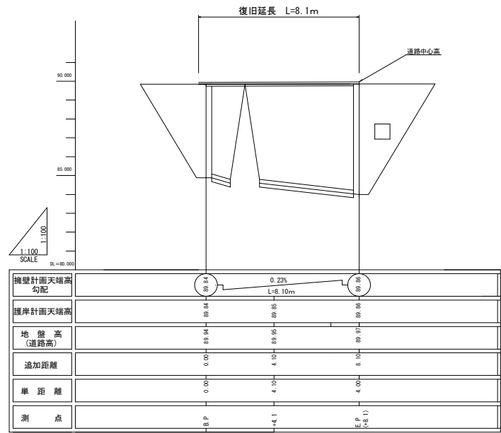
縦断面図 S=1:100
