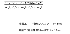
道路敷舗装 (アスファルト) S=1:10
