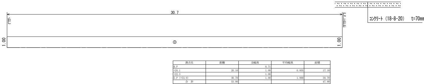
防草コンクリート 構造図 S=1:20
