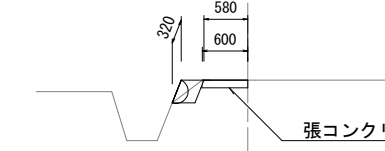
石積工(右側) 展開図 S=1:50
