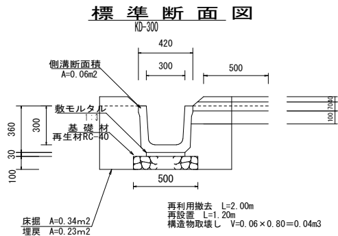
鉄筋コンクリートU形（道路用KD）数量表 10m当り
