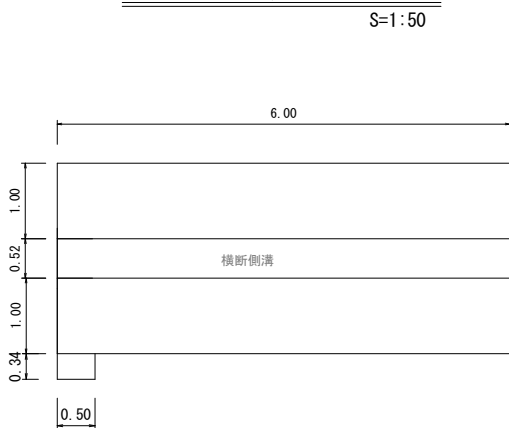
すり付け舗装 展開図
