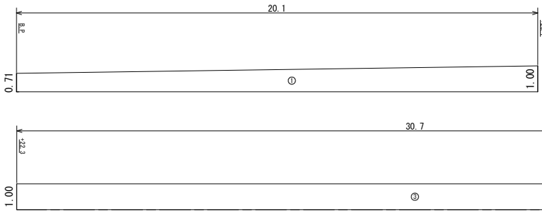
防草コンクリート工 展開図 S=1:100
