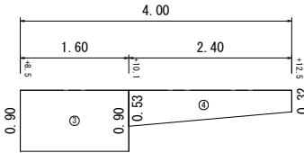
石積工(左側) 展開図 S=1:50
