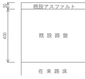
(既設舗装断面)
