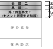
(計画舗装断面)
