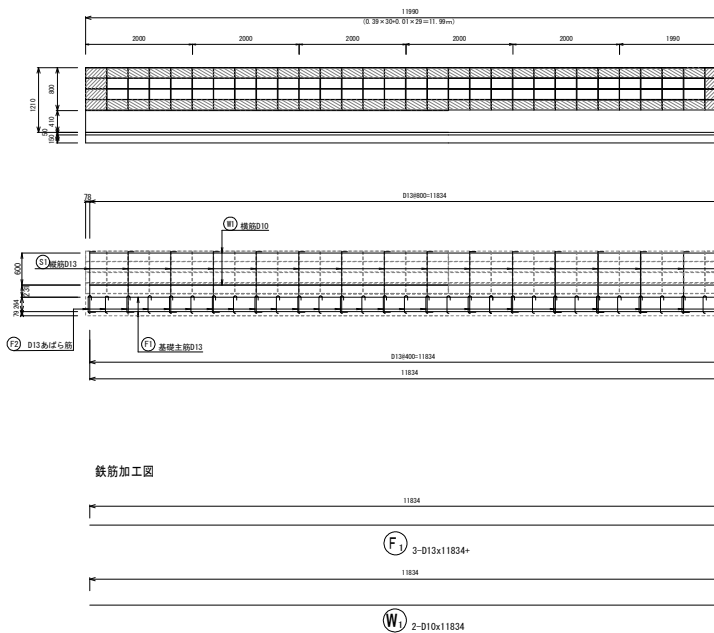
ブロック積工展開図 S=1:50
