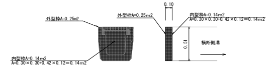
側溝改良工 構造図 S=1:20
