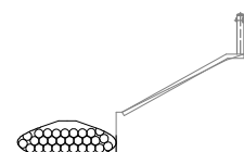
袋詰玉石 断面図 S=1:50
