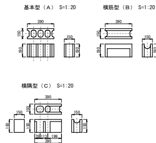
ブロック標準図
