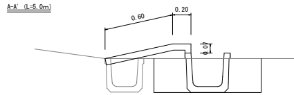
標準横断面 S=1:20
