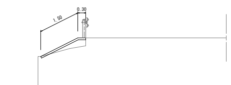
1工区 標準断面図 S=1:50
