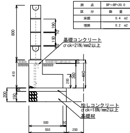
標準部断面図 S=1:20 H=800
