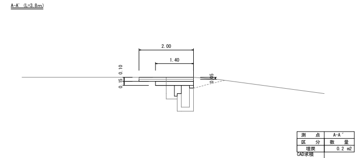
構造物取壊 展開図 S=1:50
