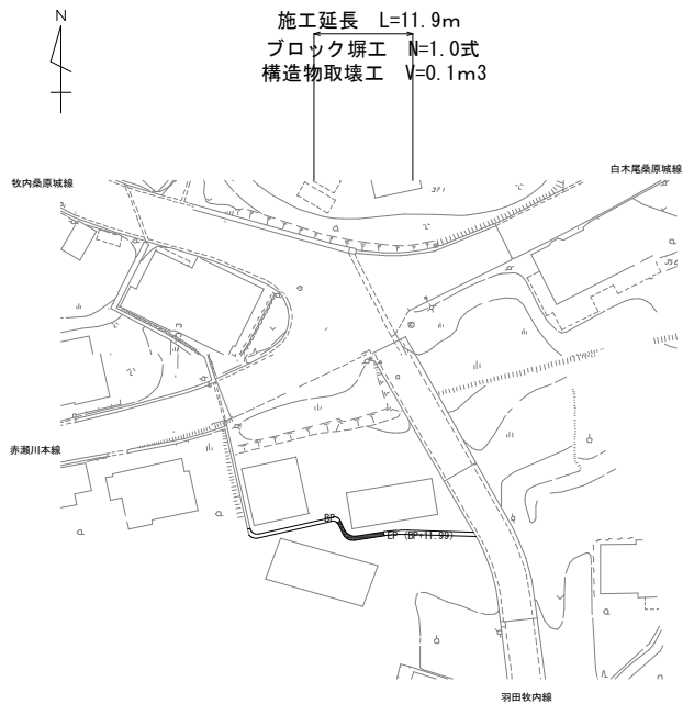
平面図 S=1:500
