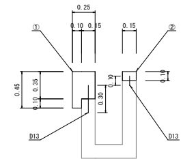
側溝改良工 構造図 S=1:20
