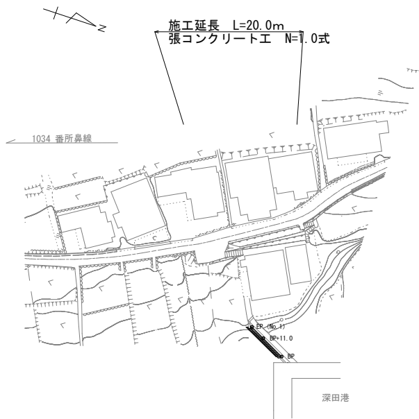
平面図 S=1:500 [番所鼻線]
