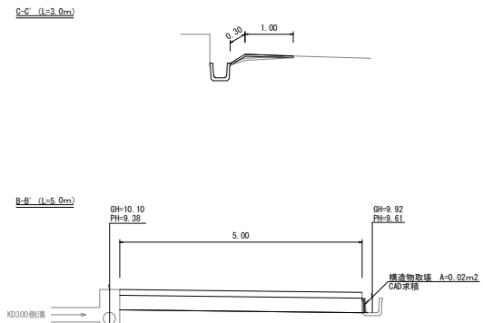
横断面 S=1:50
