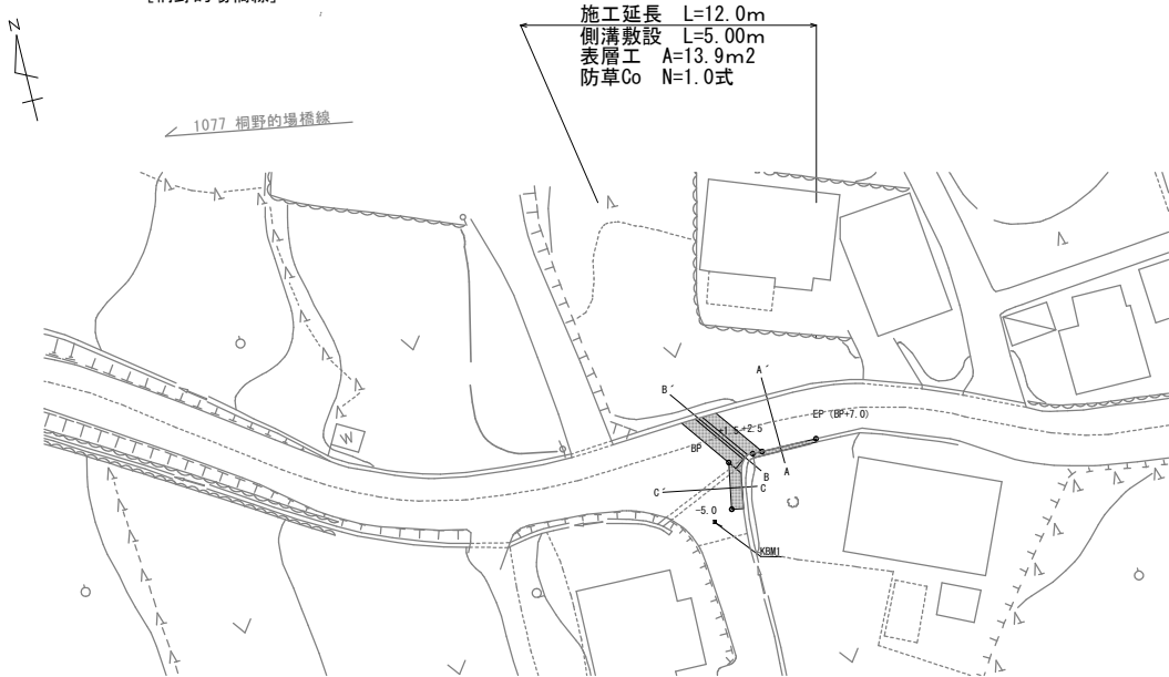
平面図 S=1:250 [桐野の場橋線]
