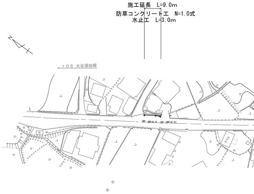
平面図 S=1:500 [大谷深田線]
