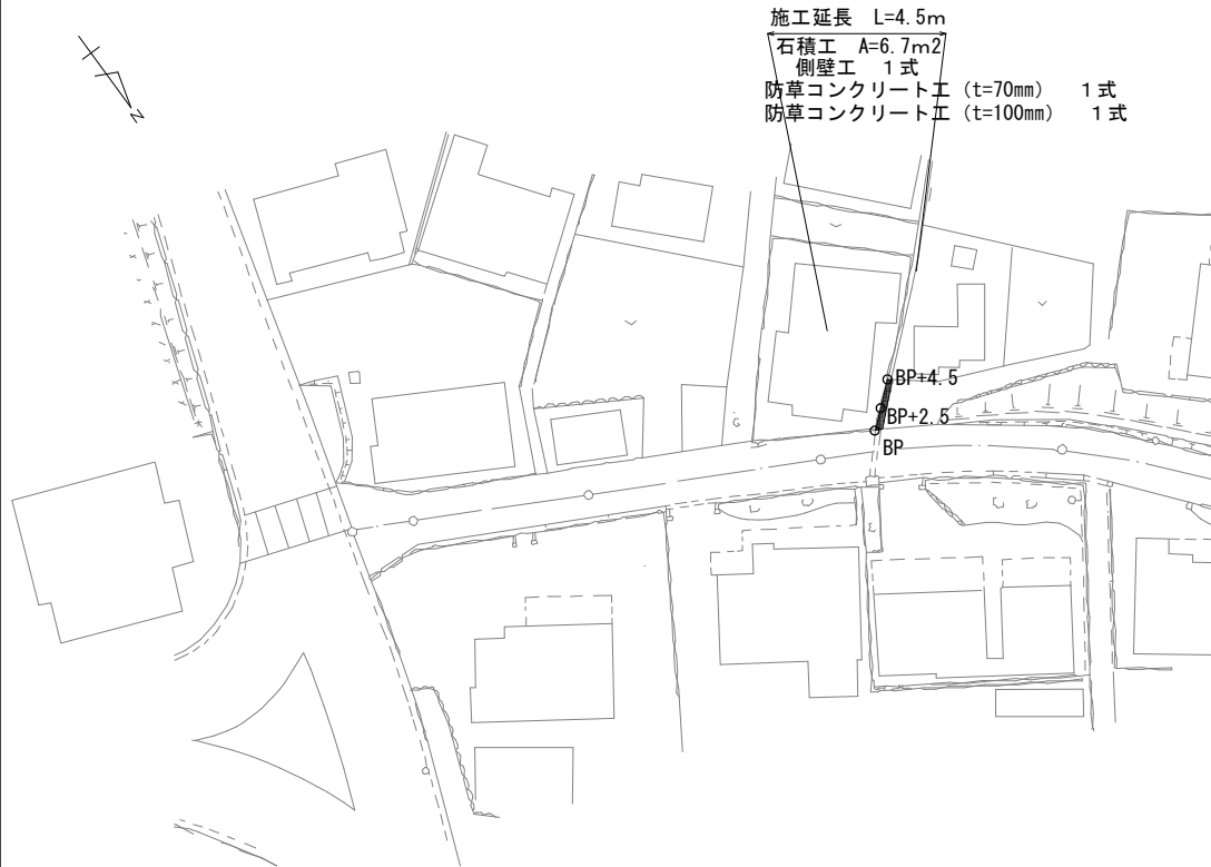
平面図 S=1:250 [岩船線]
