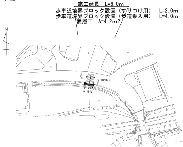
平面図 S=1:500
