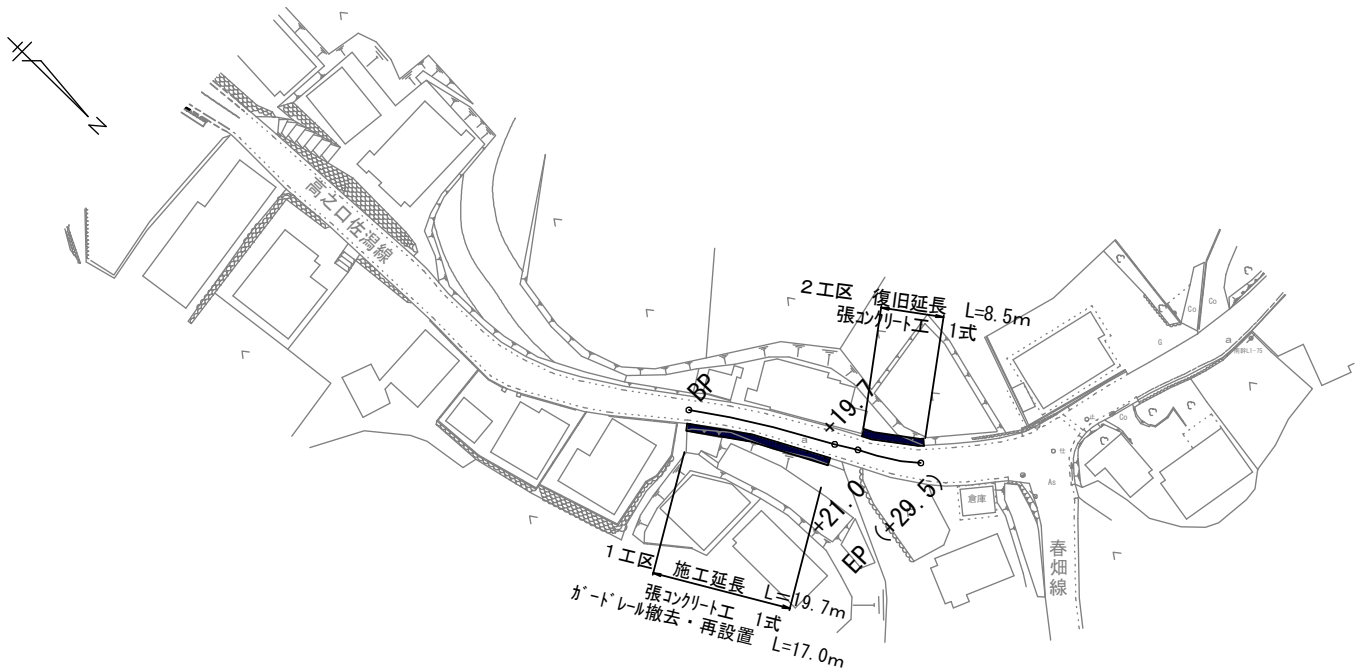
平面図 S=1:500 (市道高之口佐潟線)
