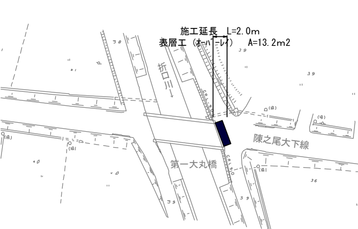
平面図 S=1:500 (市道陳之尾大下線)
