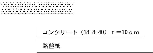
構造図 S=1:10
