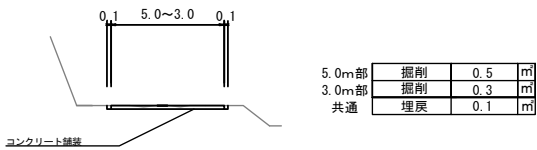
標準断面図 S=1:100
