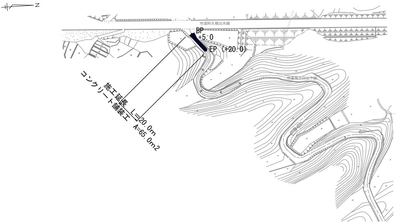
平面図 S=1:1000 (市道高之口山下線)
