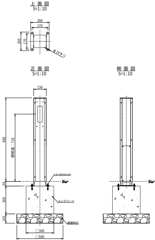
ソーラーフットライト (STFC1514R76W) 姿図
