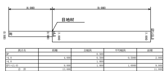
2工区 張コンクリート展開図 S=1:100
