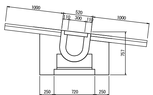
1工区 落蓋側溝横断面図 S=1:20
