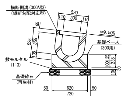
1工区 落蓋側溝断面図 S=1:20 300×300横断用
