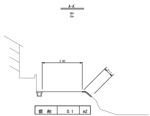
2工区 張コンクリート横断面図 S=1:100
