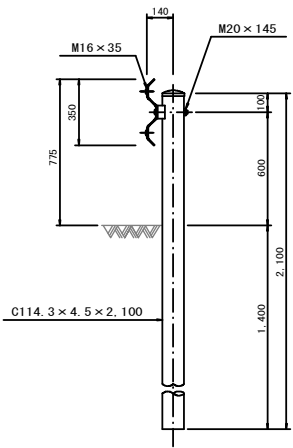
断面図 S=1:20
