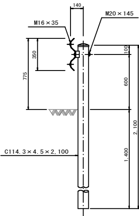
実施設計図
