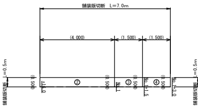
舗装工展開図 S=1:100
