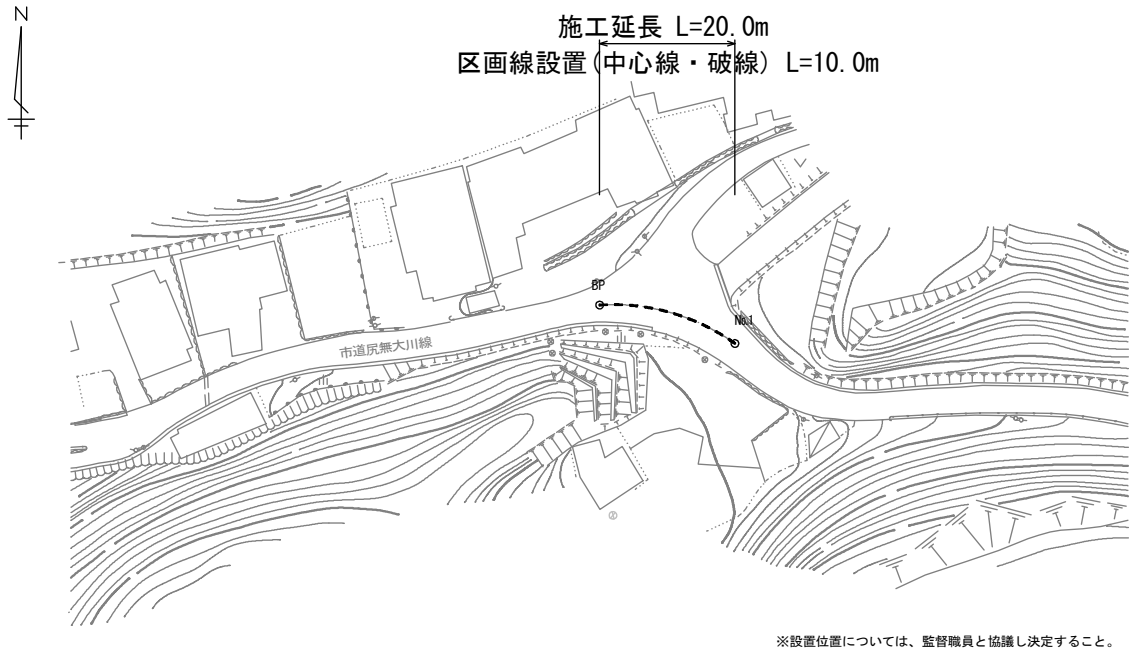
平面図 S=1:500 [尻無大川線]
