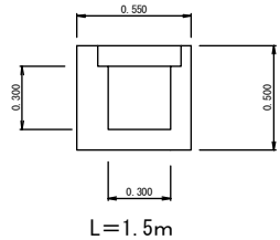
構造物取壊し S=1:20
