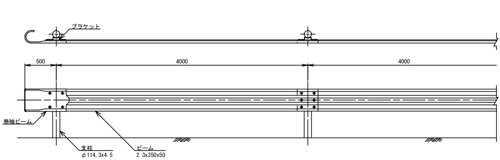
平面及び正面図 S=1:30
