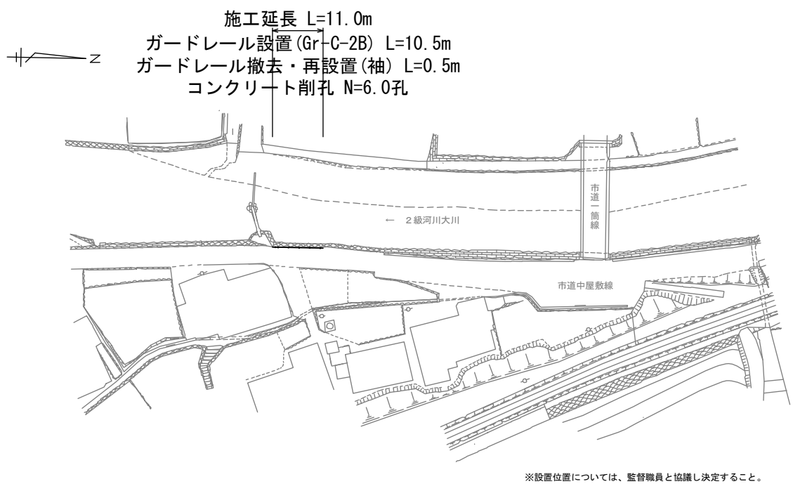
平面図 S=1:500 [中屋敷線]
