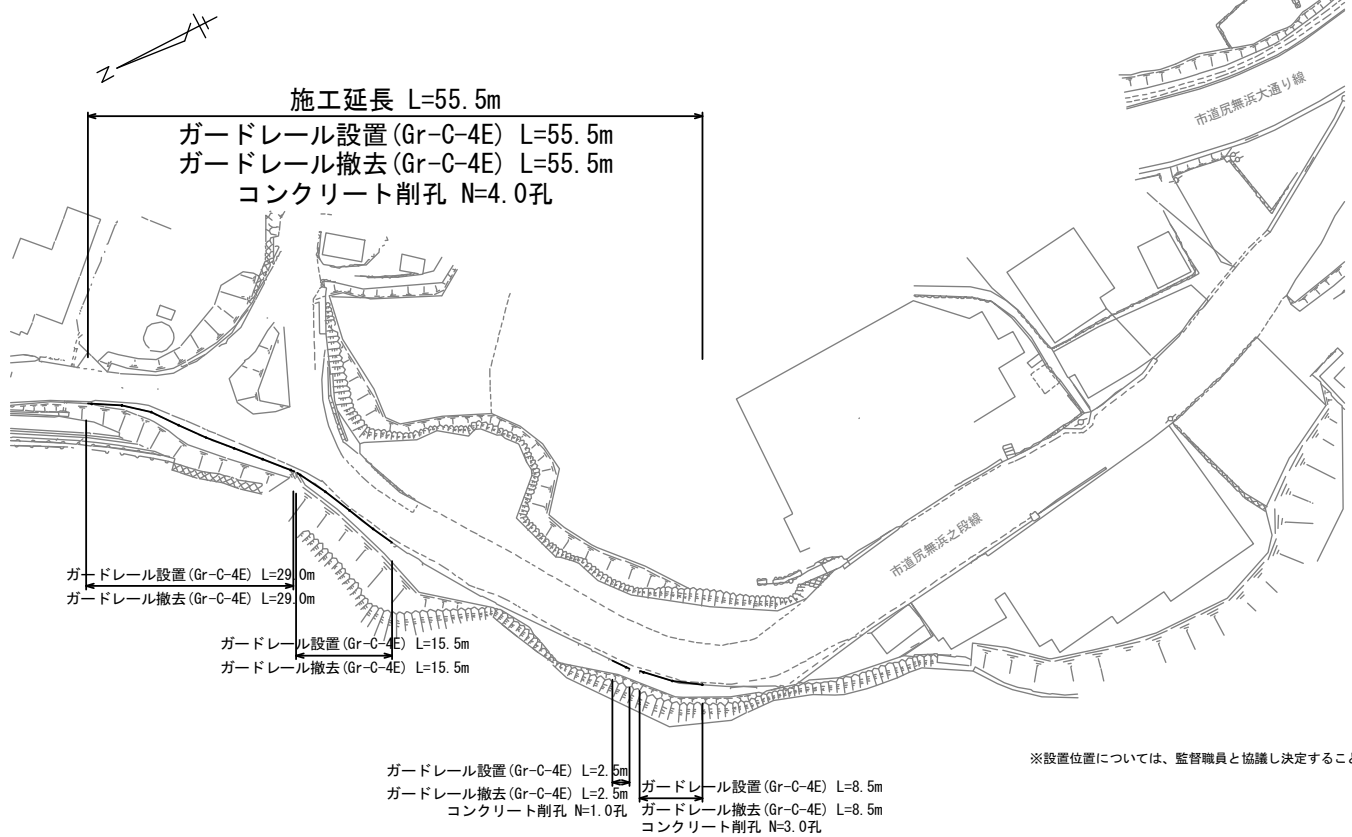
平面図 S=1:500 [尻無浜之段線]
