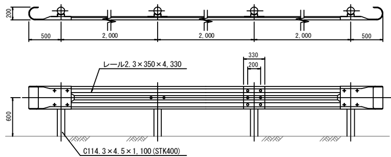
平面及び正面図 S=1:30
