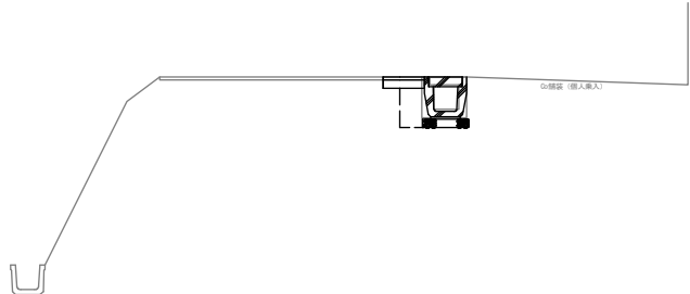
舗装工 S=1:20
