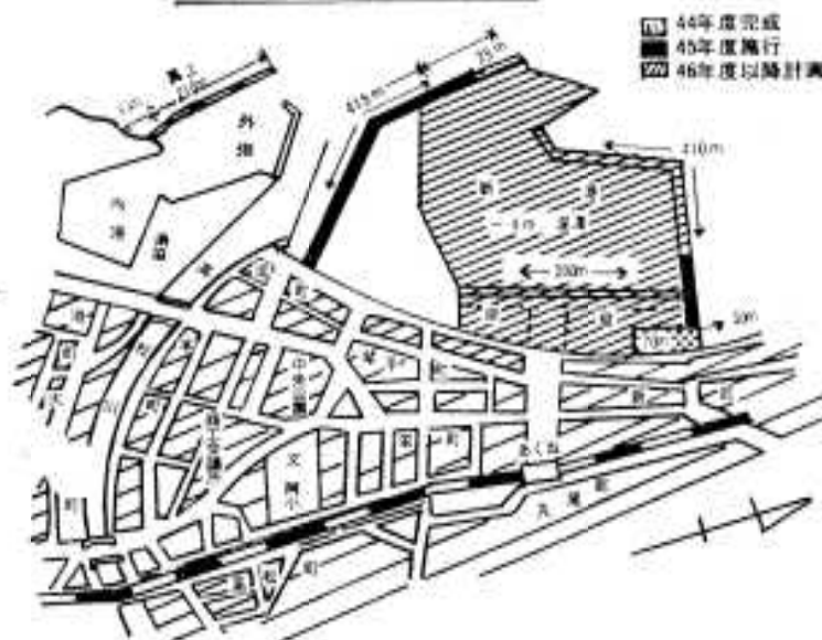
阿久根新港計画完成図
