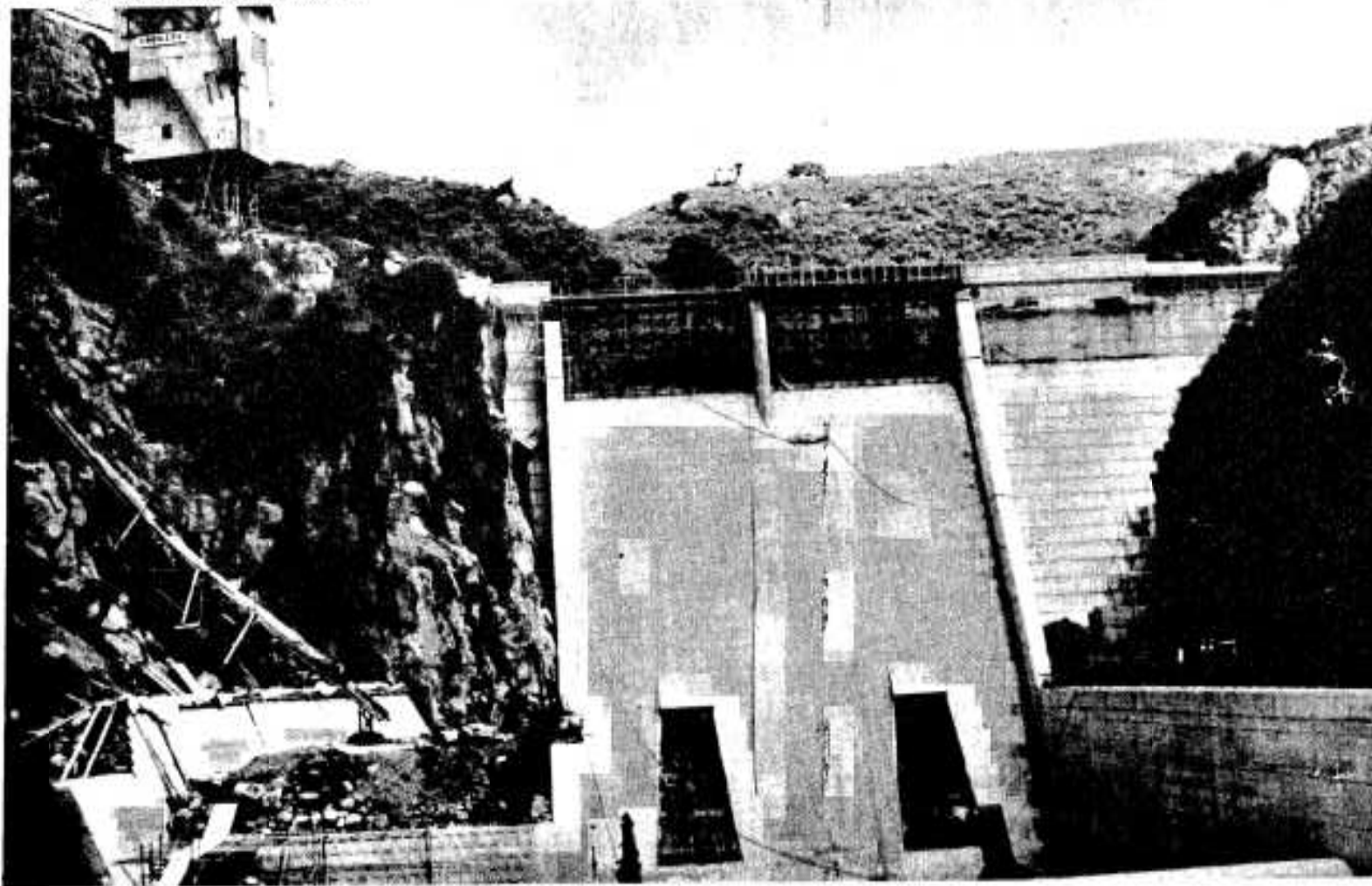
完成間近い高松川防災ダム
