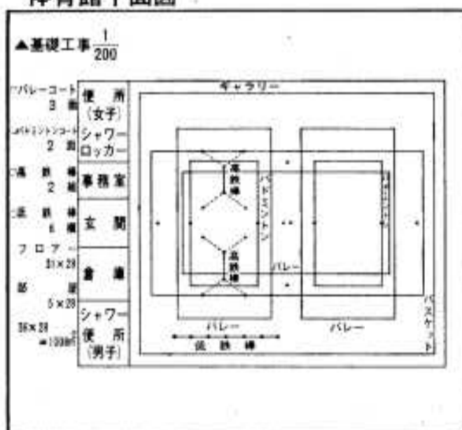
体育館平面図
