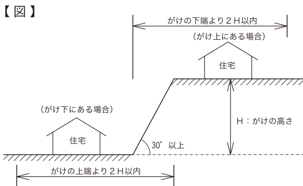
※がけに近接している住宅とは、上図のとおり2H以内にある住宅のことです。
