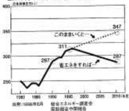
■2010年までの日本のCO 2 排出量推計
