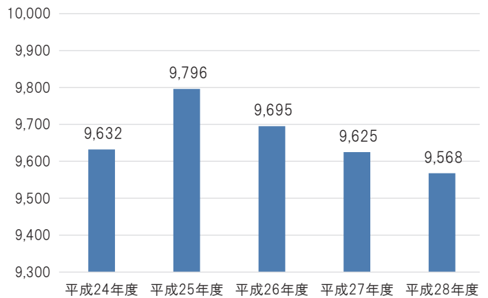
市債現在高の推移
