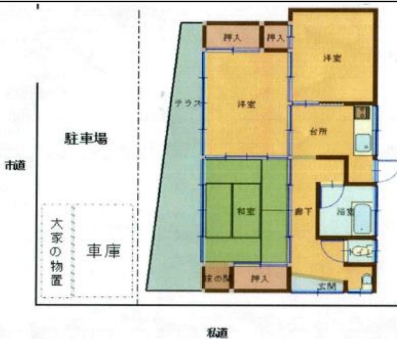
間取り図（赤瀬川3891-3）
